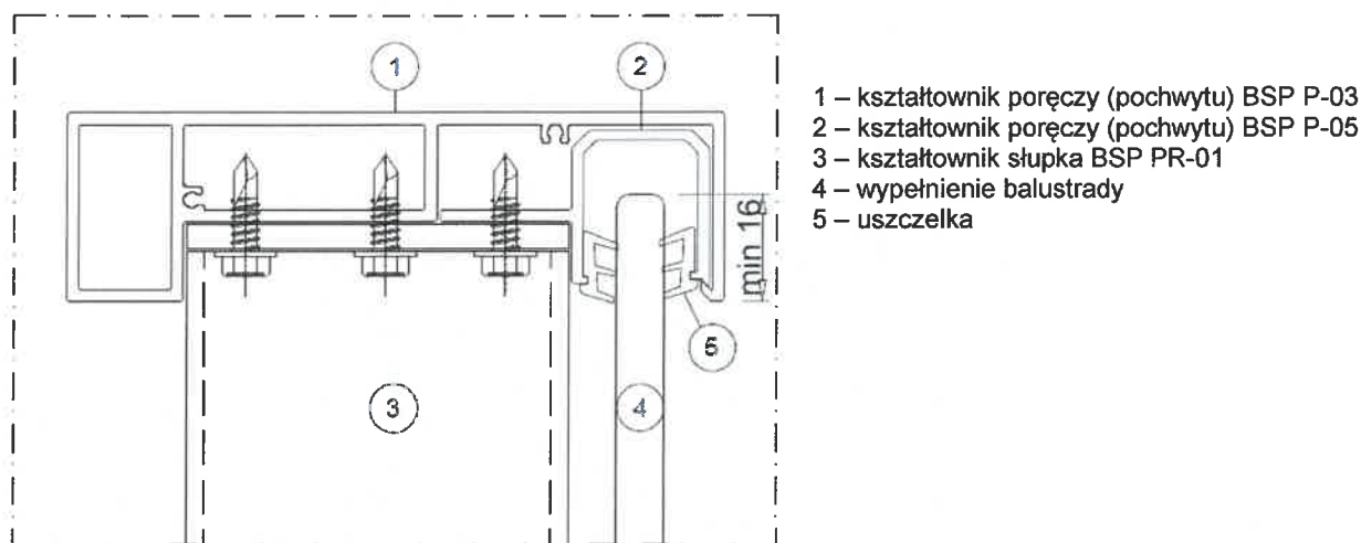
Rysunek C25. Detal poręczy (pochwyty) dwuczęściowego (wymiary w mm)
