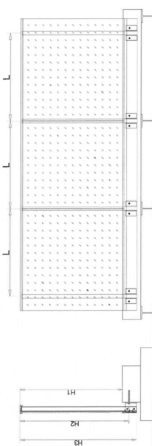
Rysunek D2. Widok balustrady BSP KB, oznaczenie wysokości H1, H2 i H3 – odmiana BSP KB-SZ-B ze szkłem ESG VSG
