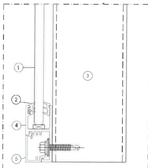
Rysunek C17. Detal połączenia wypełnienia z modułów fotowoltaicznych ze słupkiem
