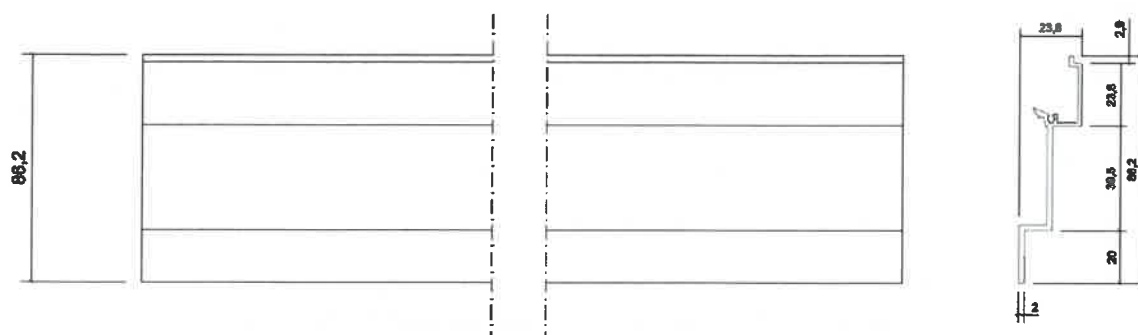
Rysunek B11. Kształtownik do zamocowania maskownicy BSP MP-01
