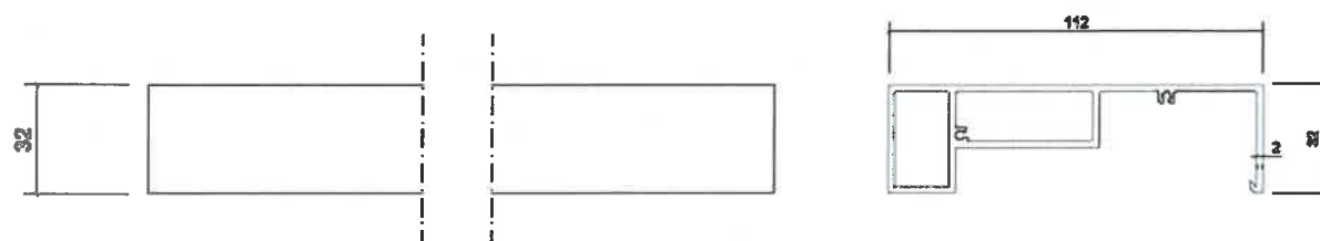
Rysunek B8. Kształtownik poręczy (pochwyty) BSP P-03
