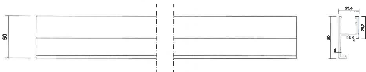
Rysunek B5. Kształtownik mocujący wypełnienie BSP MS-01-G
