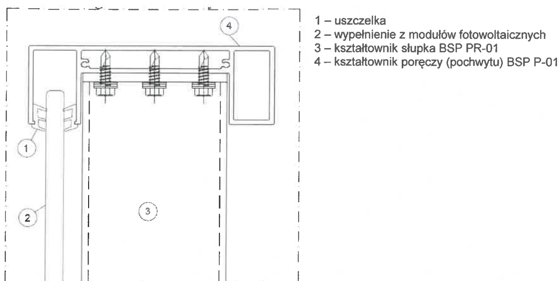
Rysunek C22. Detal połączenia wypełnienia z modułów fotowoltaicznych z poręczą (pochwytem)
