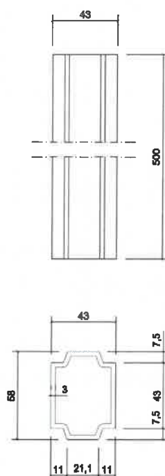
Rysunek B13. Kształtownik wzmocnienia słupka BSP WZ-01
