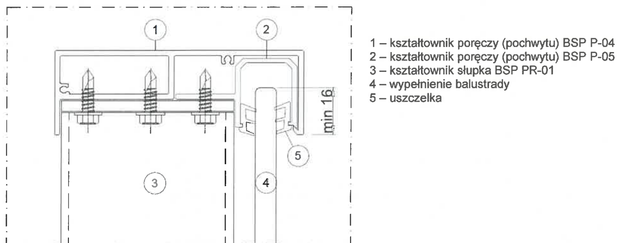
Rysunek C26. Detal poręczy (pochwyty) dwuczęściowego (wymiary w mm)
