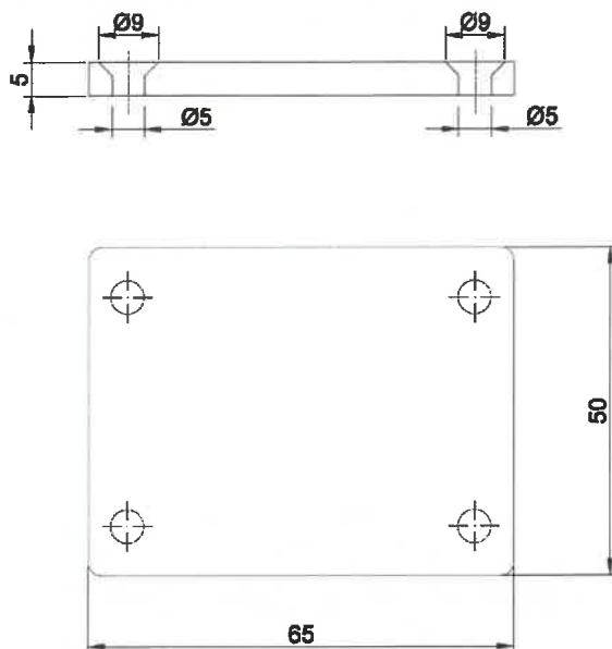
Rysunek B20. Zaślepka kształtownika słupka BSP PR-01
