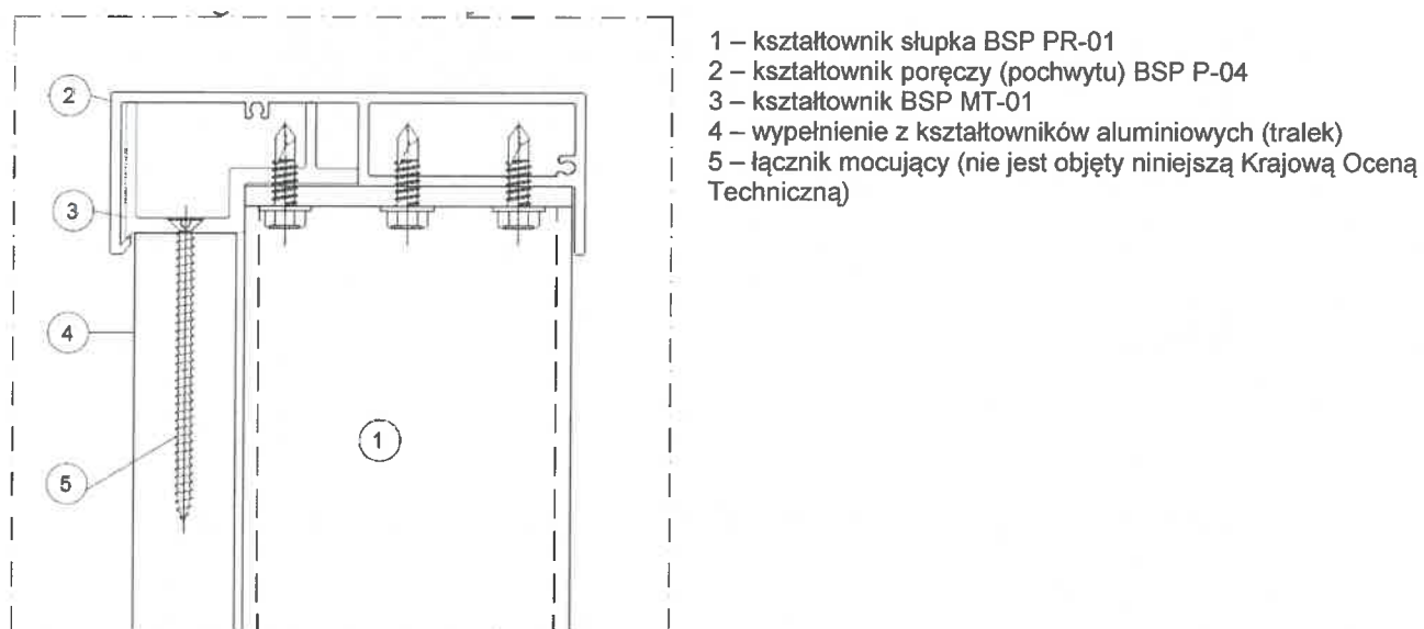
Rysunek C23. Detal połączenia wypełnienia z kształtowników aluminiowych (tralek) z poręczą (pochwytem)
