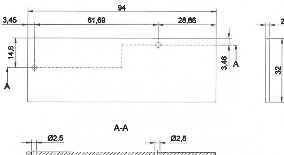
Rysunek B19. Zaślepka kształtowników poręczy (pochwyty) BSP P-04 BSP P-05
