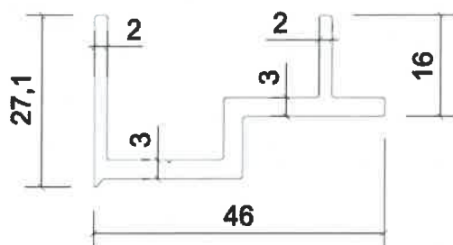
Rysunek B14. Kształtownik BSP MT-01 – kształtownik górny mocujący wypełnienie z pionowych kształtowników aluminiowych (tralek) i wypełnienie z blachy perforowanej aluminiowej
