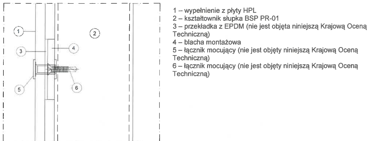
Rysunek C24. Detal połączenia wypełnienia z płyty HPL z kształtownikiem słupka, w połowie wysokości wypełnienia
