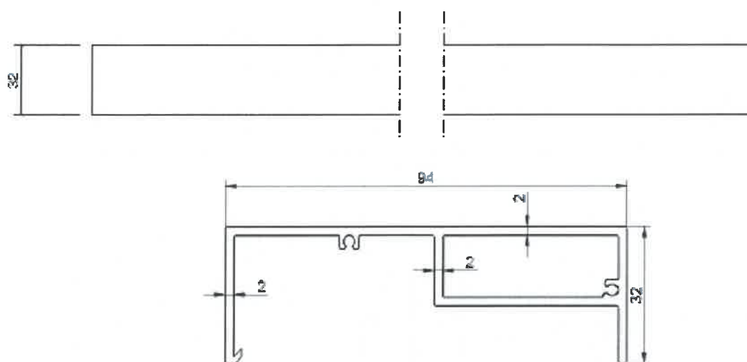
Rysunek B9. Kształtownik poręczy (pochwyty) BSP P-04
