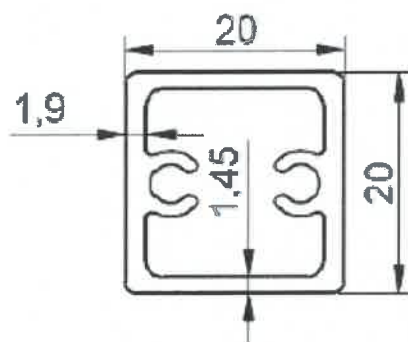
Rysunek B22. Kształtownik tralki BSP TR-01
