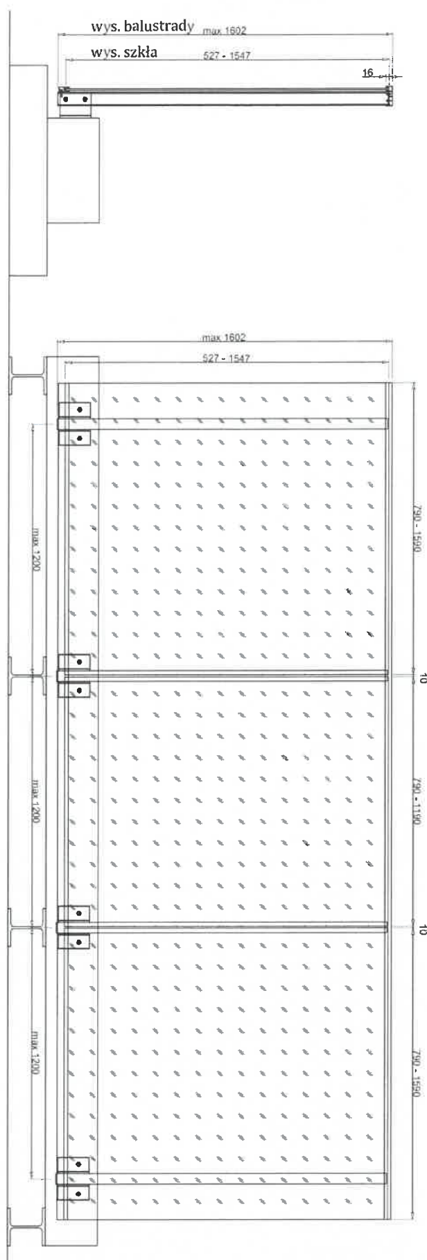
Rysunek C1. Balustrada odmiany BSP KB-SZ ze szkłem VSG – widok i przekrój pionowy
