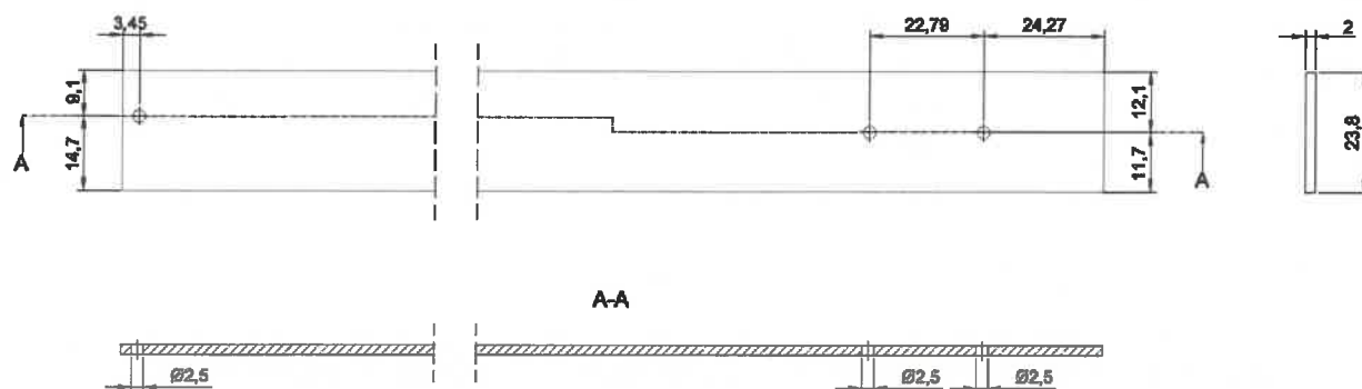
Rysunek B17. Zaślepka kształtowników do zamocowania maskownicy BSP MP-01 i BSP MP-02
