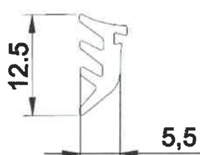
285N uszczelka górna i dolna do szkła 44.2
