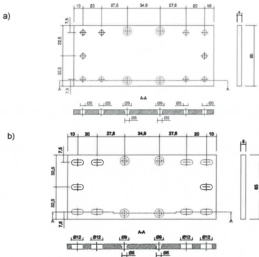
Rysunek B16. Blacha montażowa poręczy (pochwyty) a) z otworami stałymi, b) z otworami przesuwными
