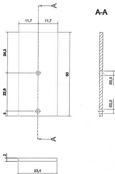
Rysunek B18. Zaślepka kształtowników mocujących wypełnienie BSP MS-01 i BSP MS-02
