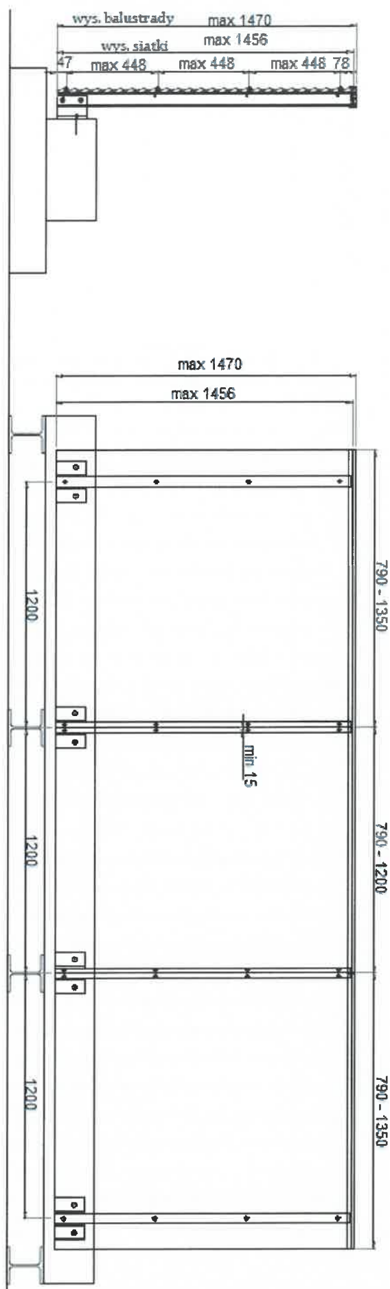
Rysunek C7. Balustrada odmiany BSP KB-CC – widok i przekrój pionowy
