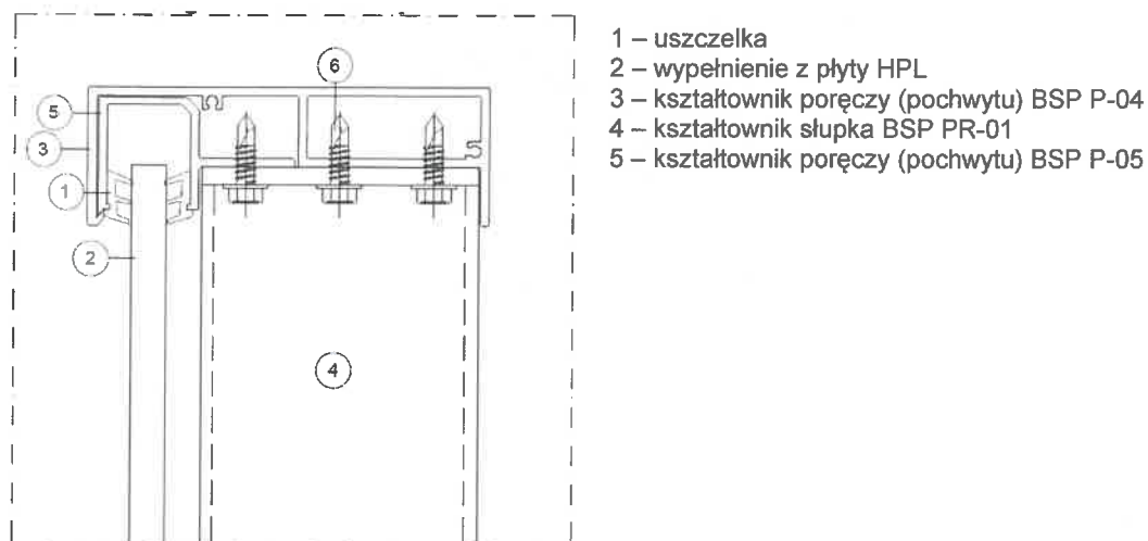
Rysunek C21. Detal połączenia wypełnienia z płyty HPL z poręczą (pochwytem)
