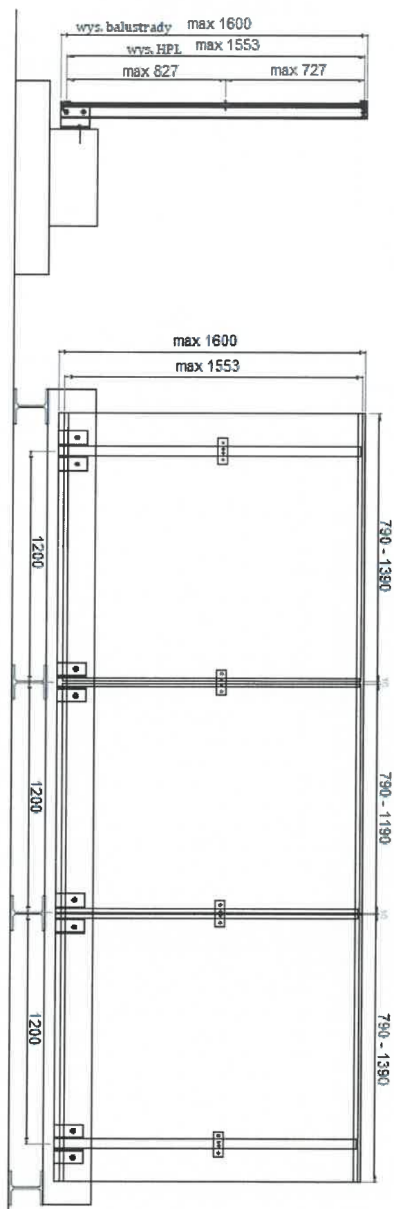
Rysunek C6. Balustrada odmiany BSP KB-HP – widok i przekrój pionowy
