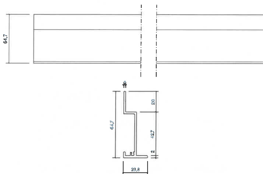
Rysunek B12. Kształtownik do zamocowania maskownicy BSP MP-02
