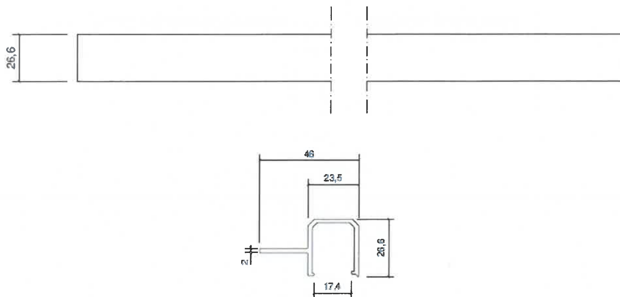
Rysunek B10. Kształtownik poręczy (pochwyty) BSP P-05
