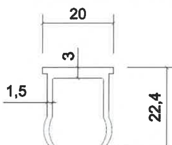
Rysunek B15. Kształtownik BSP MT-02 – kształtownik dolny mocujący wypełnienie z pionowych kształtowników aluminiowych (tralek)
