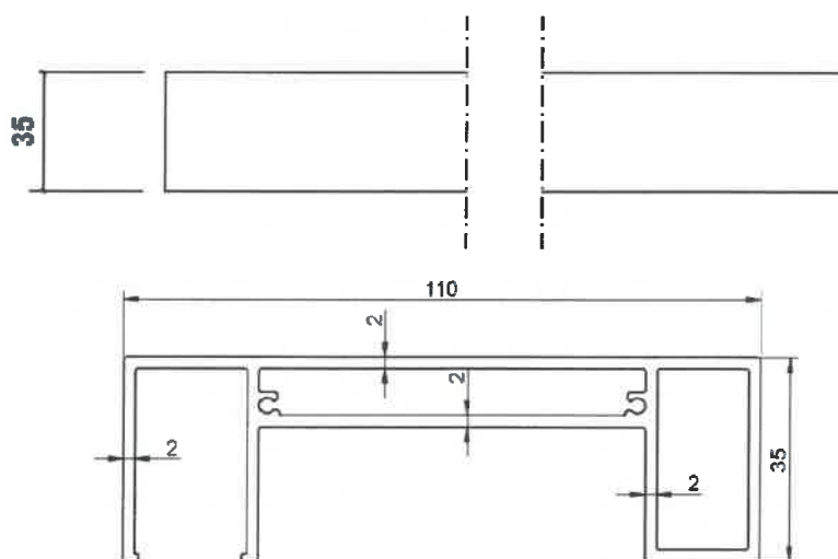
Rysunek B6. Kształtownik aluminiowy do wykończenia kształtownika mocującego wypełnienie BSP MS-02
