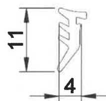
289N uszczelka górna i dolna do szkła 55.2
