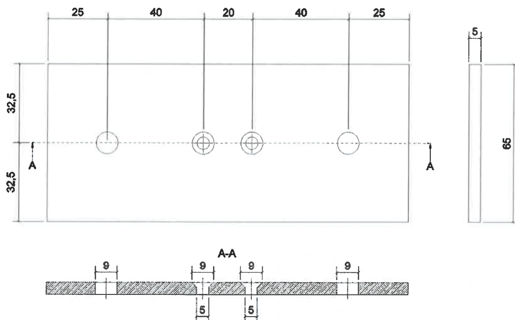
Rysunek B23. Blacha montażowa do mocowania wypełnienia z płyt HPL
