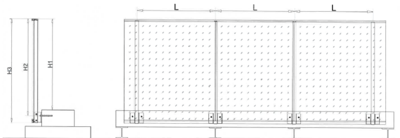
Rysunek D2: Balustrada odmiany KB-SZ-B
