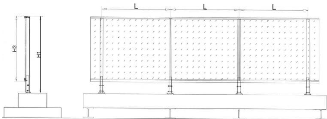
Rysunek D3: Balustrada odmiany KBS-SZ
