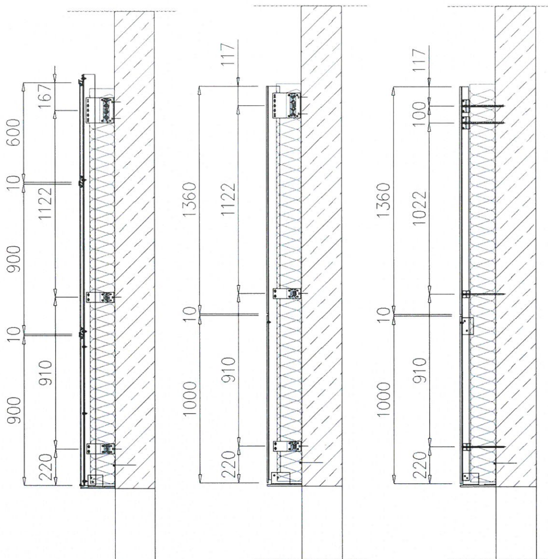
Rys. 12. Przekroje P1 (po lewej), P2 (w środku) i P3 (po prawej)
