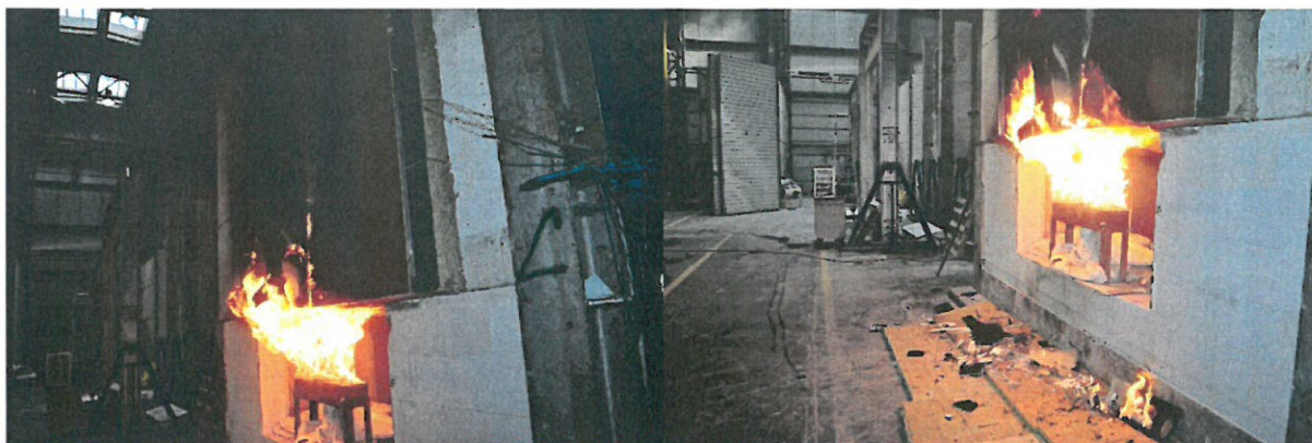
Rys. 19. Widok próbki podczas badania – 12 minuta
