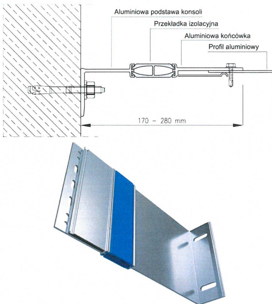
Rys. 5. Schemat montażu i budowy oraz wizualizacja konsoli BSP KW4 PAS
