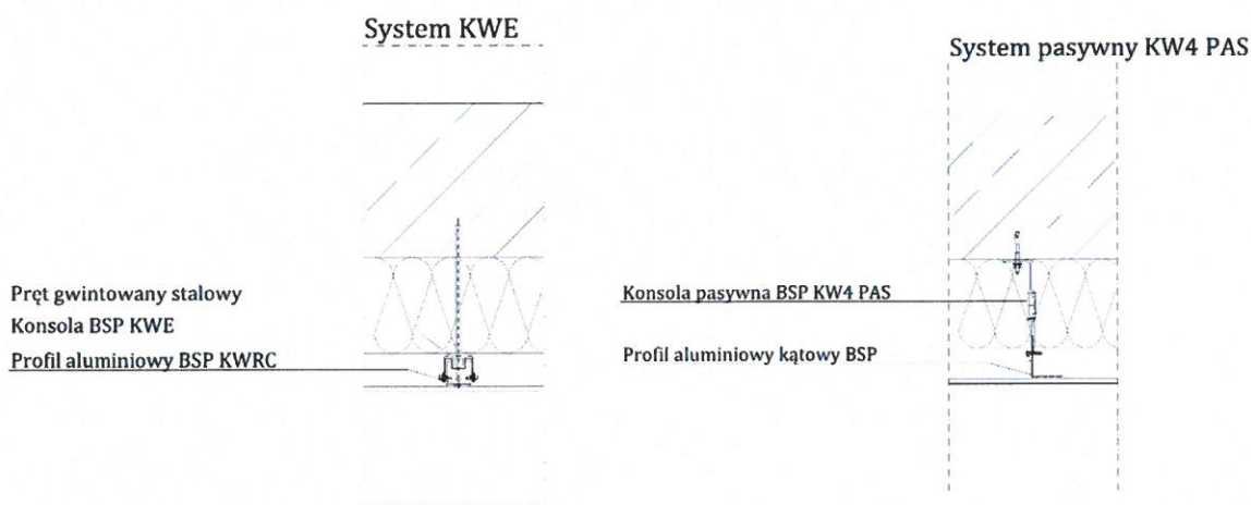
Rys. 1. Detal mocowania - system KWE, profil KWRP (po lewej) i system KW4 PAS
