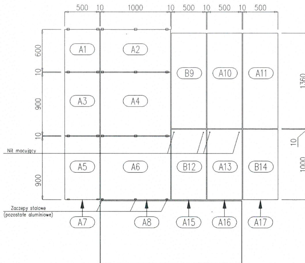
Rys. 9. Widok – układ płyt, oznaczenie płyt
