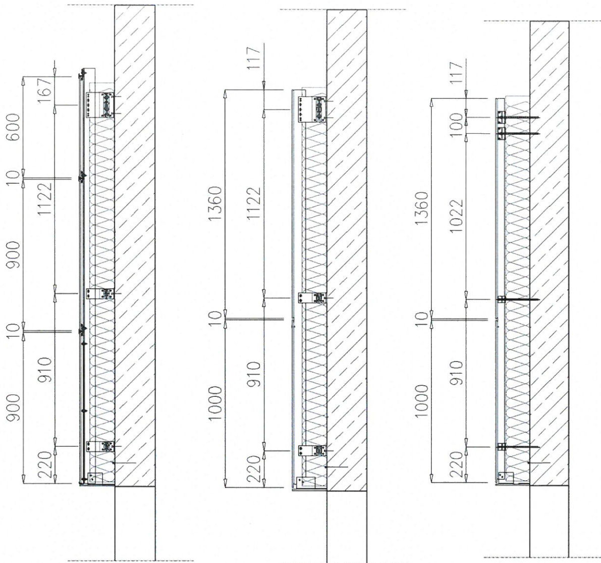
Rys. 12. Przekroje P1 (po lewej), P2 (w środku) i P3 (po prawej)
