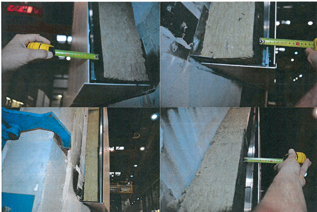
Rys. 14. Widok gotowej próbki przed rozpoczęciem badania - detale.
