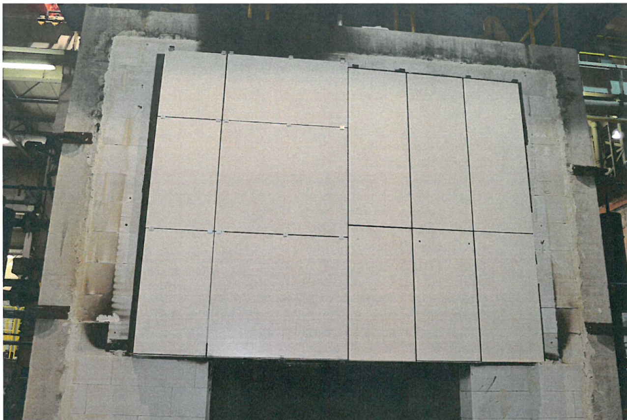
Rys. 13. Widok gotowej próbki przed rozpoczęciem badania.
