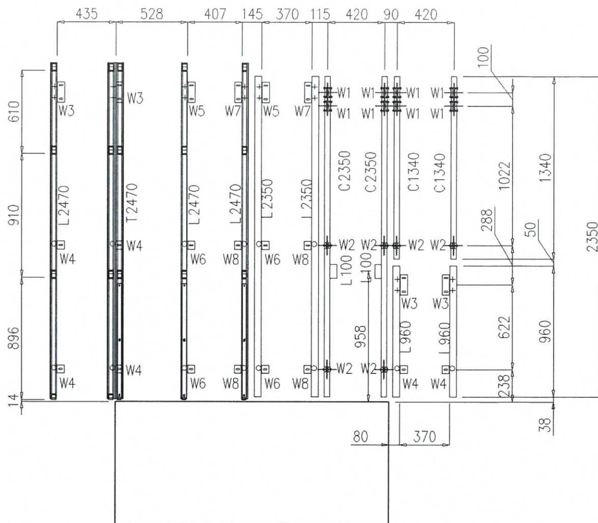
Rys. 8. Widok – układ podkonstrukcji
