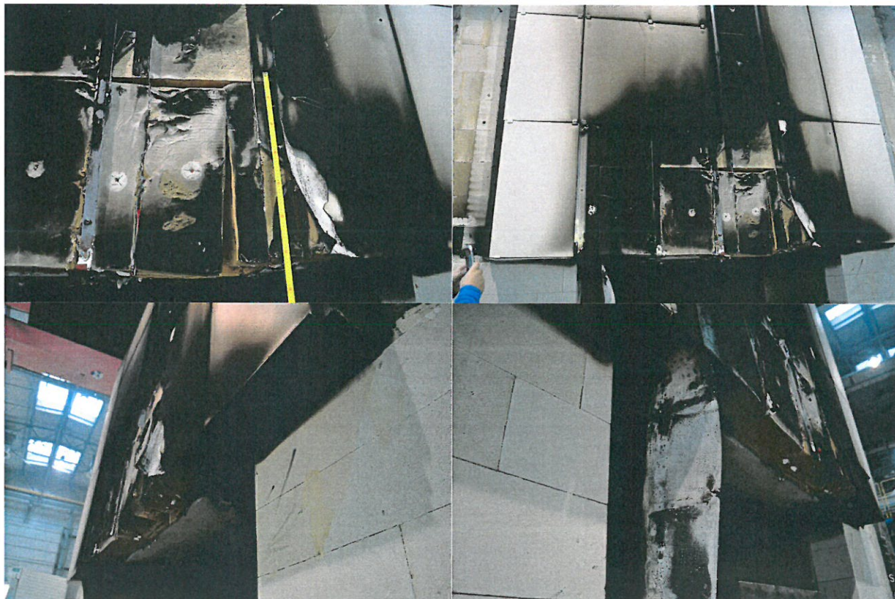
Rys. 26. Widok próbki po badaniu - detale
