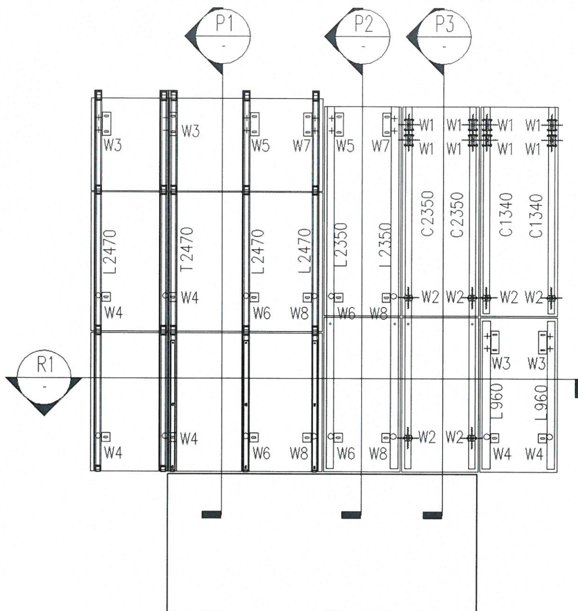
Rys. 10. Widok – układ podkonstrukcji i płyt
