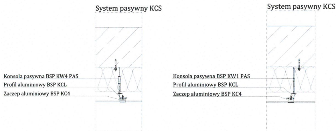
Rys. 3. Detal mocowania - system KCS, profil KCL z konsolą KW4 PAS oraz konsolą KW1 PAS
