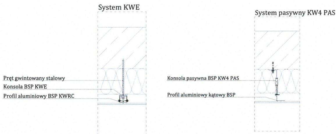
Rys. 1. Detal mocowania - system KWE, profil KWRC (po lewej) i system KW4 PAS
